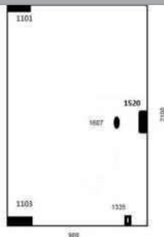
GIR-90 Porta Giro Padrao 900x2100
