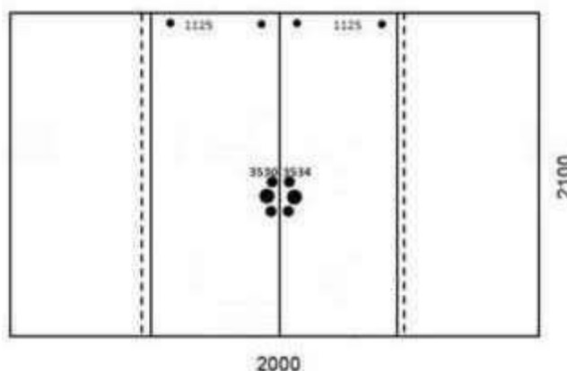
COR-2000 Porta De Correr Padrão 2000x2100 (2 Fix-050 / 2 Por-055)
